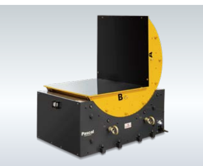
金型反転機
