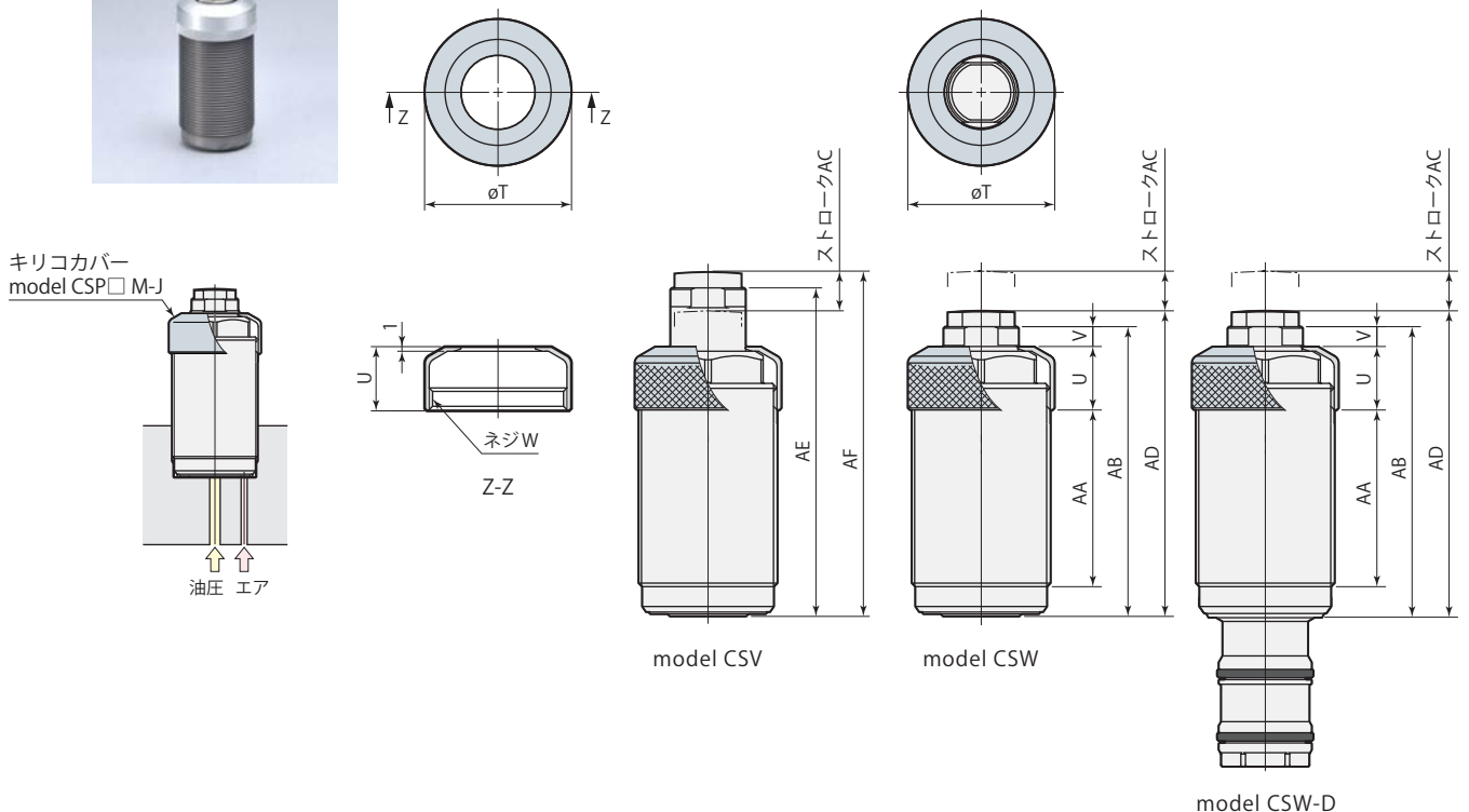
ワークサポート取付寸法
