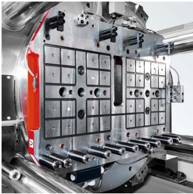
可动盘
