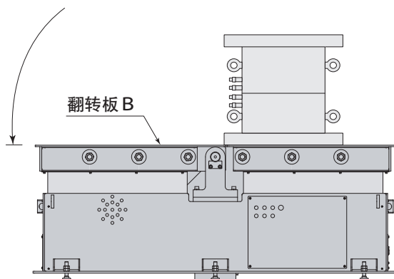
③ 翻转完了, 翻转台B收回。
