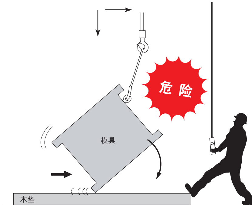
吊车要横向及纵向同时操作
