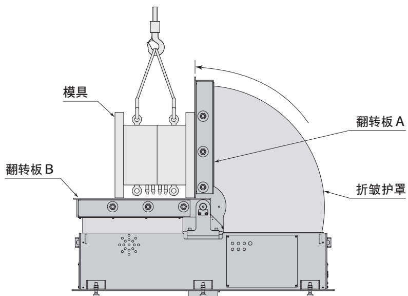
① 翻转板A立起, 搭载模具
