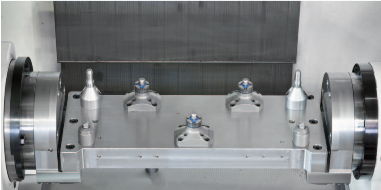
실린더헤드 가공 치구
