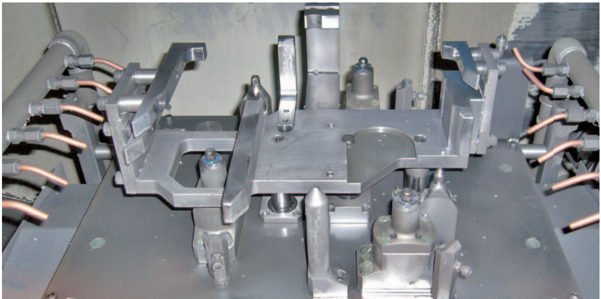
미션케이스 가공 치구
