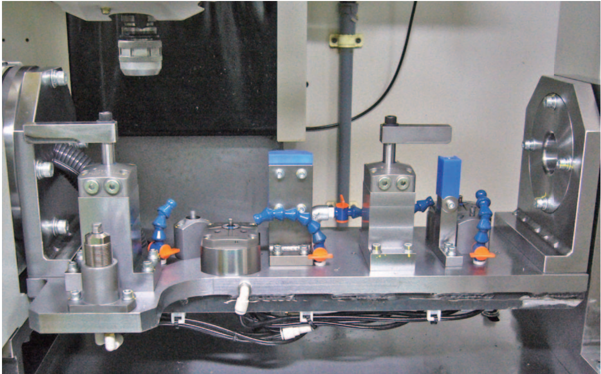
엔진부품 가공치구
