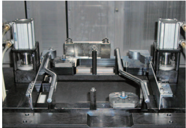
리테이너 세척 치구
