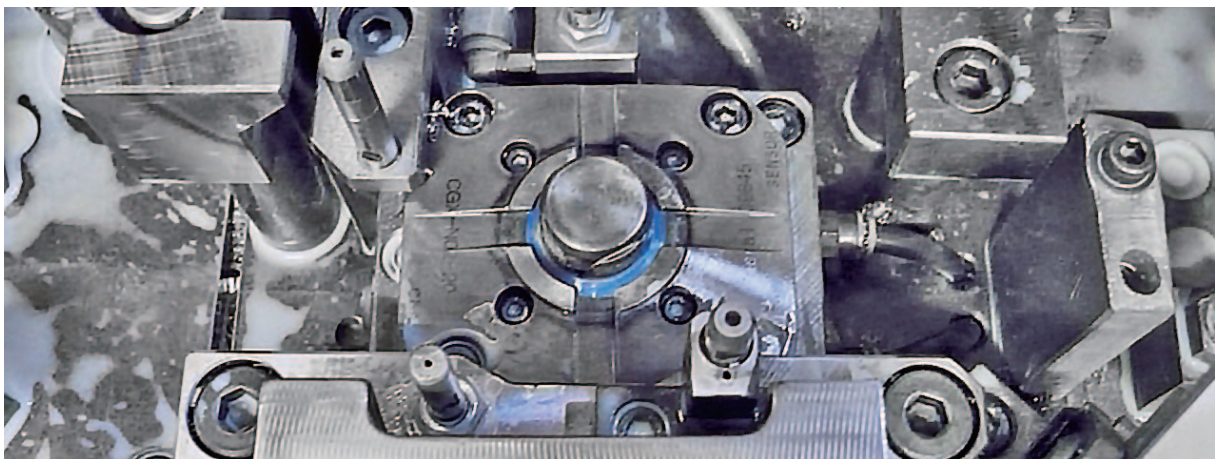
펌프커버 가공치구
