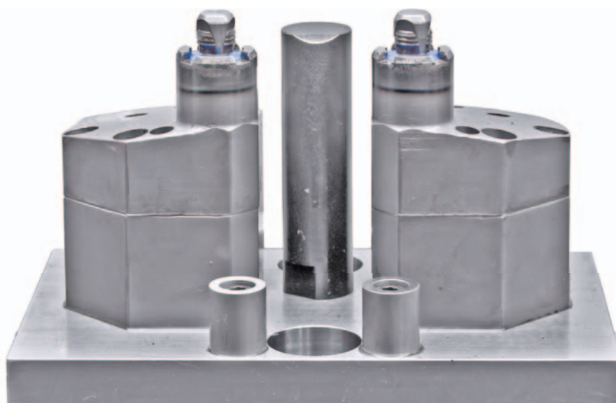
스테인리스부품 가공치구
