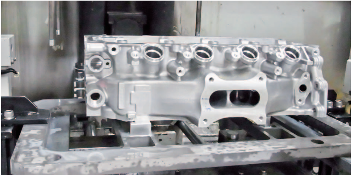
실린더 헤드
