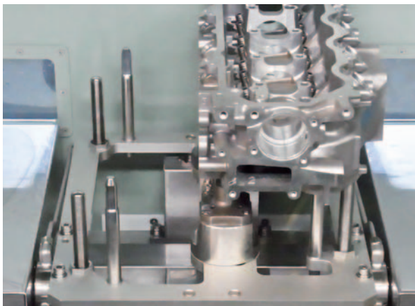
실린더헤드 세척치구
