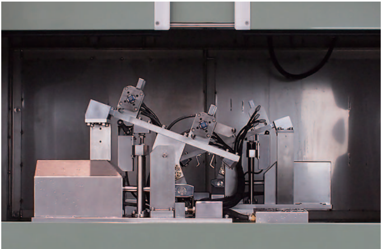
로봇세척기 치구
