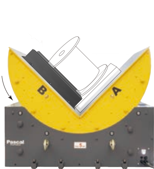
② 电缆盘翻转
