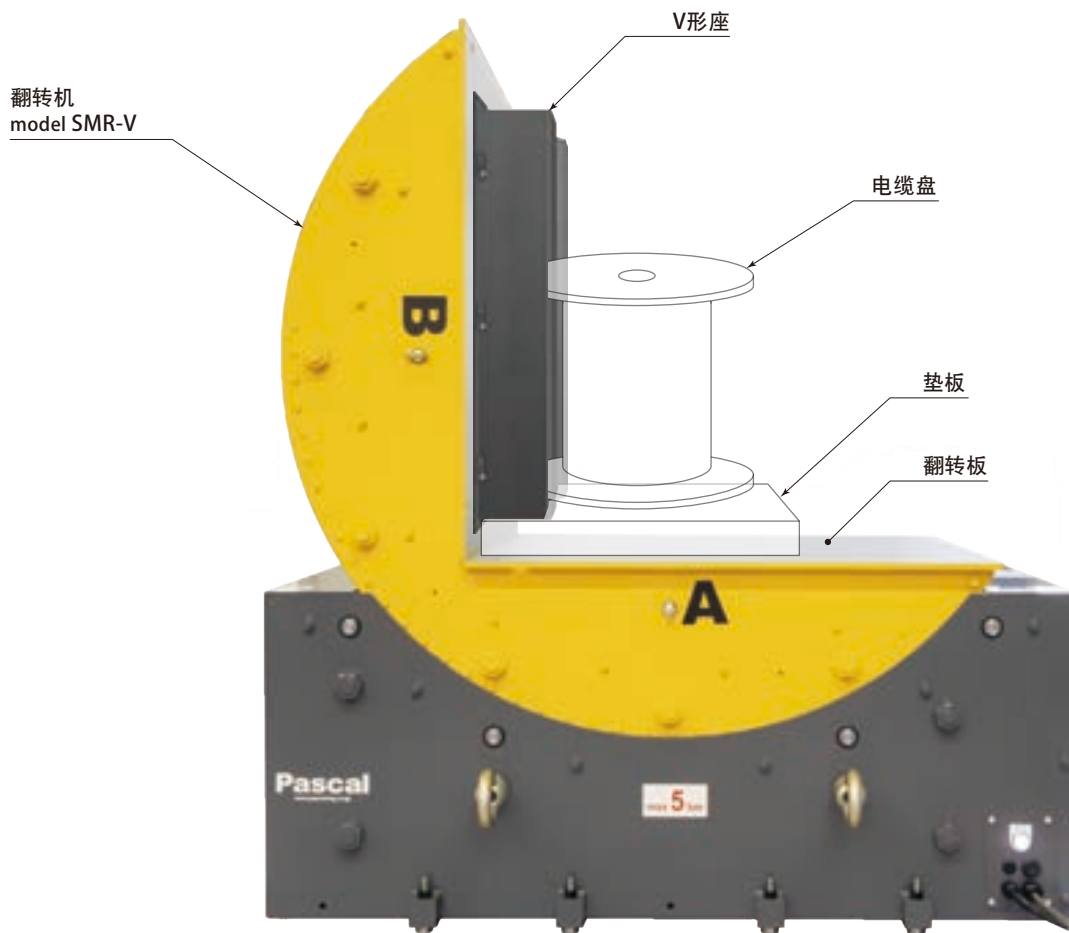
① 电缆盘设置
