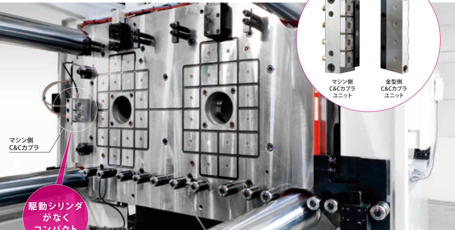
2,500kN (250ton) 2色成形機 横入れ マグクランプ 固定側 & C&Cカプラ
