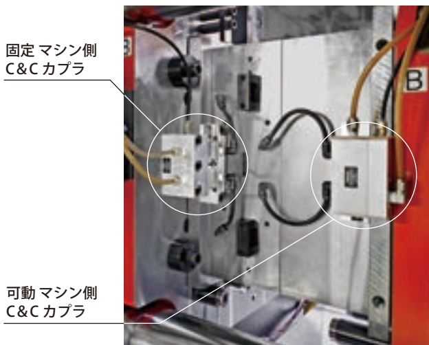
2,500kN(250ton)2色成形機 横入れ マグクランプ & C&Cカブラ
