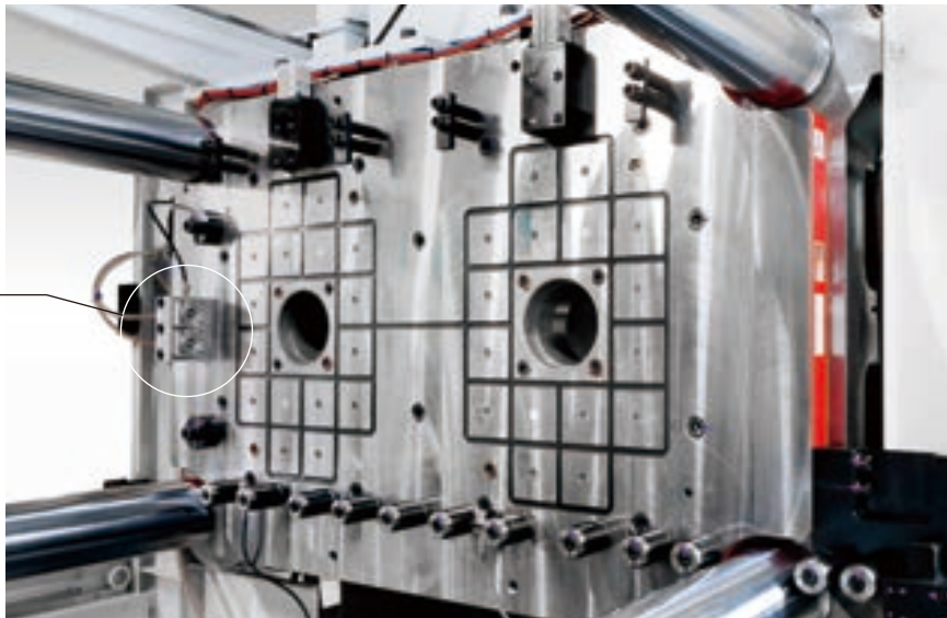
2,500kN(250ton)2色成形機 横入れ マグクランプ 固定側 & C&Cカブラ
