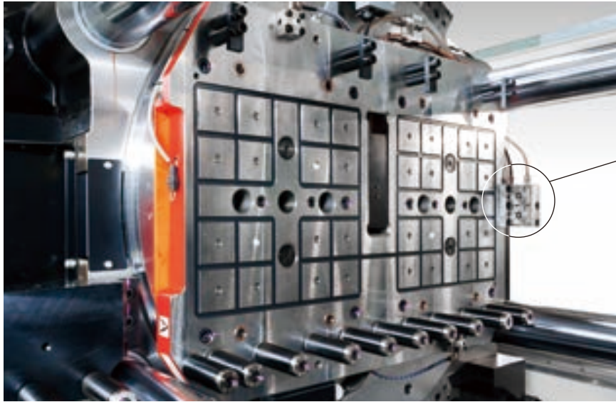
2,500kN(250ton)2色成形機 横入れ マグクランプ 可動側 & C&Cカブラ
