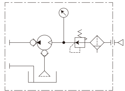
油空圧回路図
