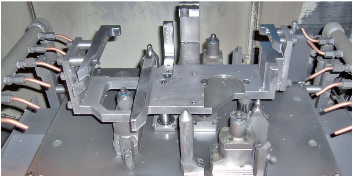
变速箱体加工夹具
