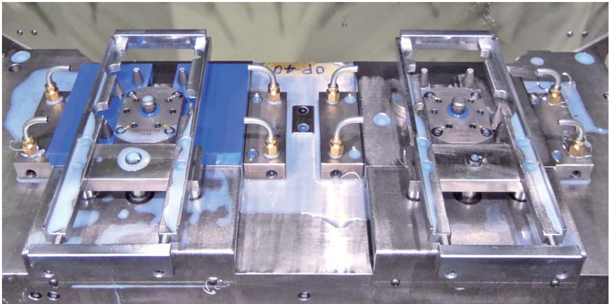
夹具组合
