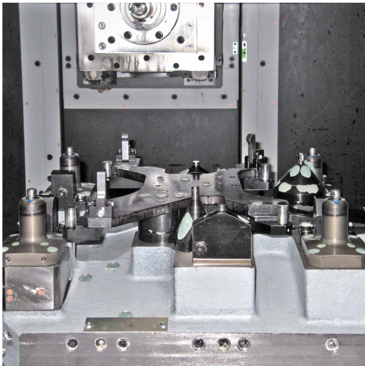
油泵加工夹具
