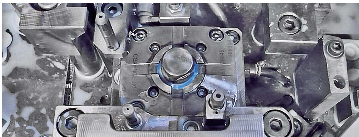
泵盖加工夹具
