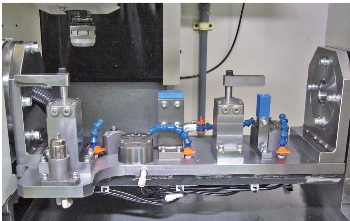
发动机部件加工夹具
