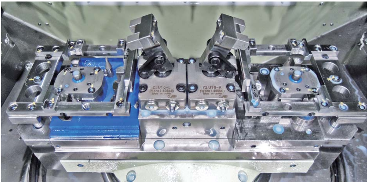
夹具组合
