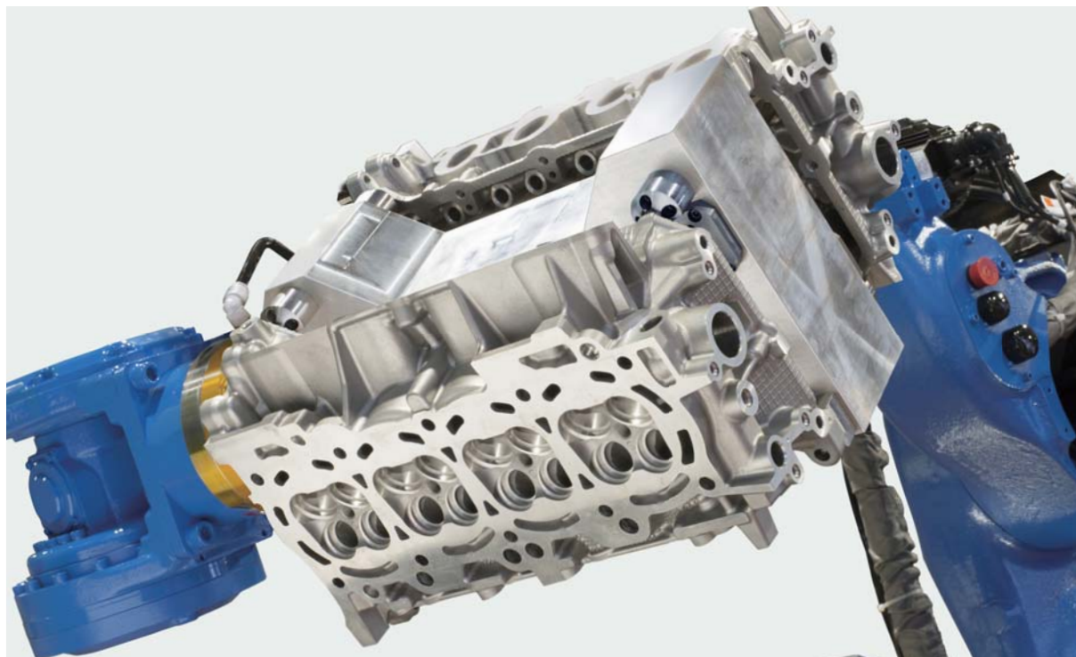
气缸盖搬送夹具
