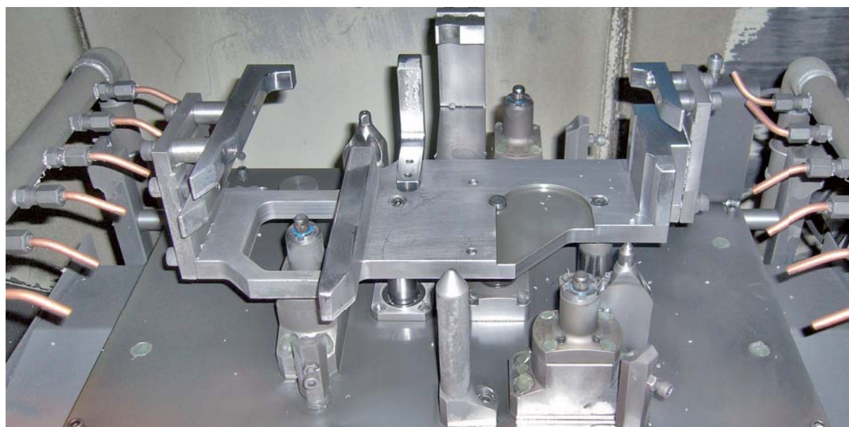
ミッションケース加工ジグ
