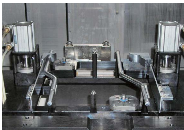
リテーナ洗浄ジグ
