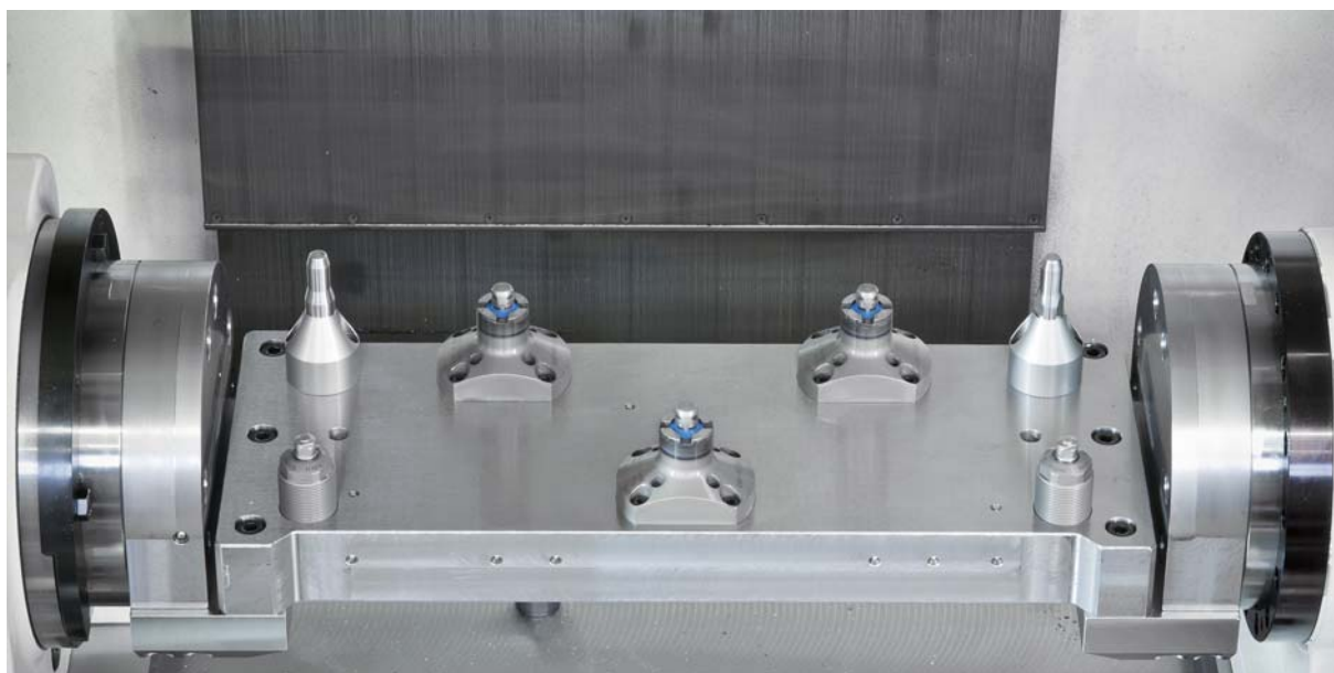
シリンダヘッド加工ジグ
