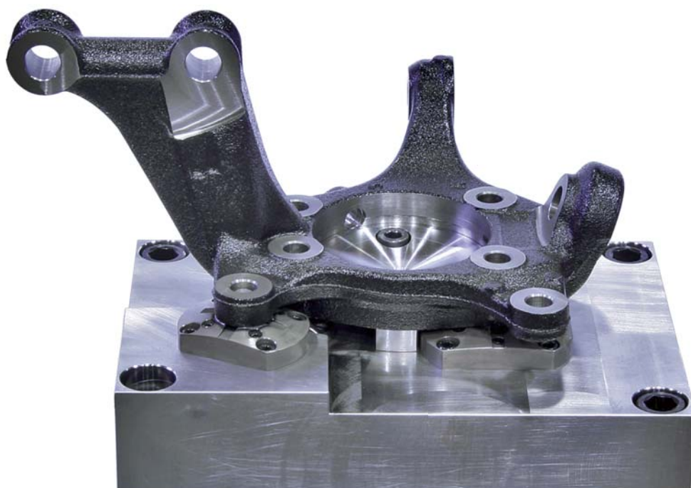
ステアリングナックル
