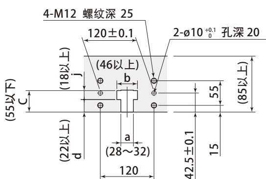
安装加工图
