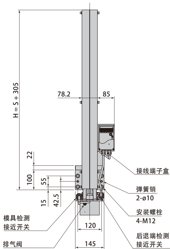
安装加工图
