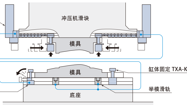
下模 旋转式夹紧器 THB
