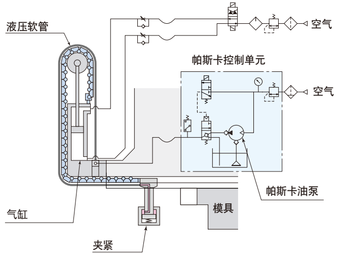
气液压回路图
