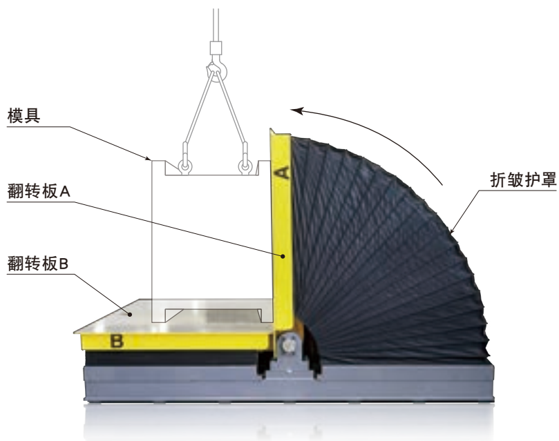
① 翻转板A立起, 搭载模具
