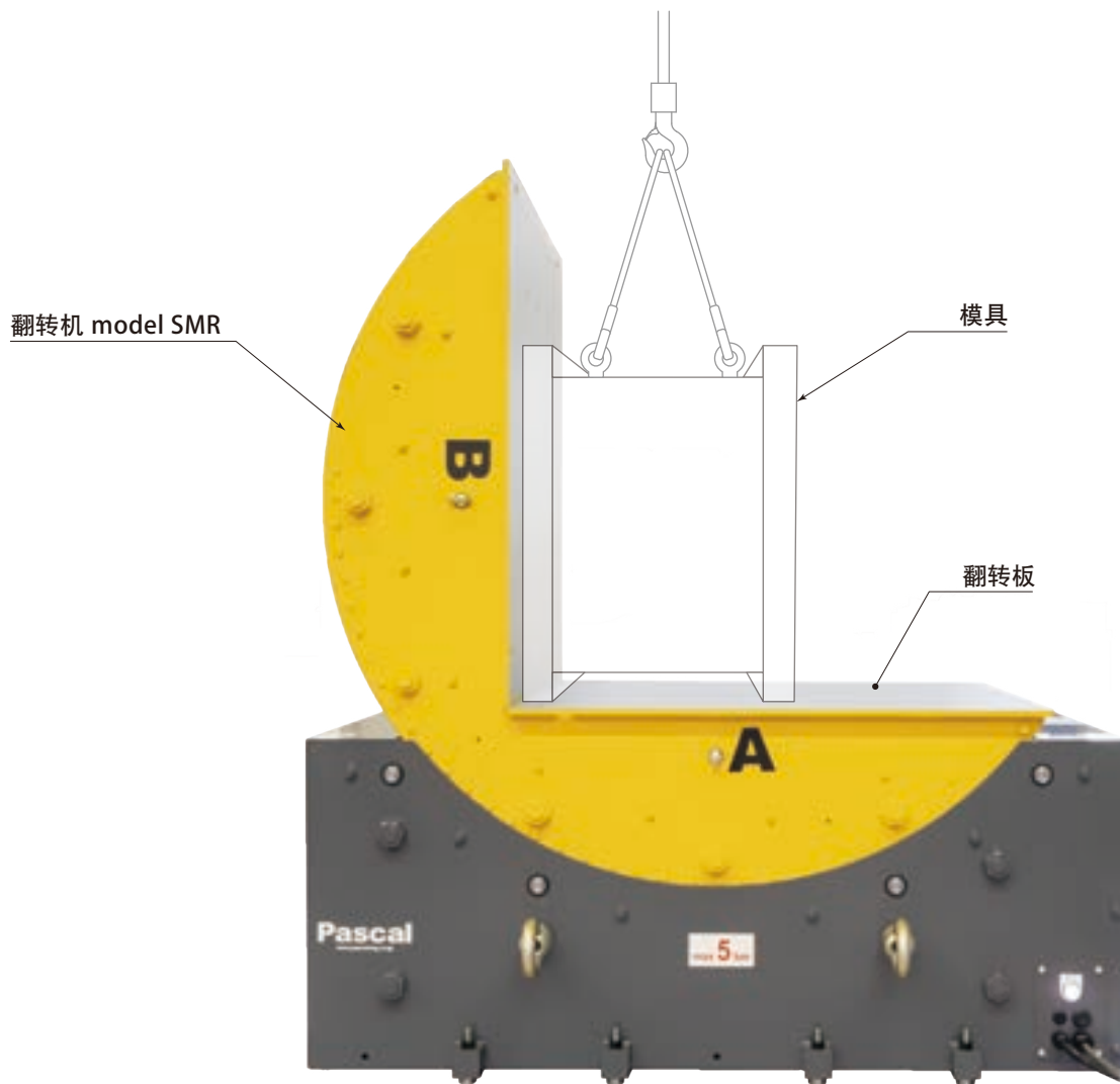
① 搭载模具
