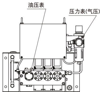
控制单元 HCSD-H2EDDD
