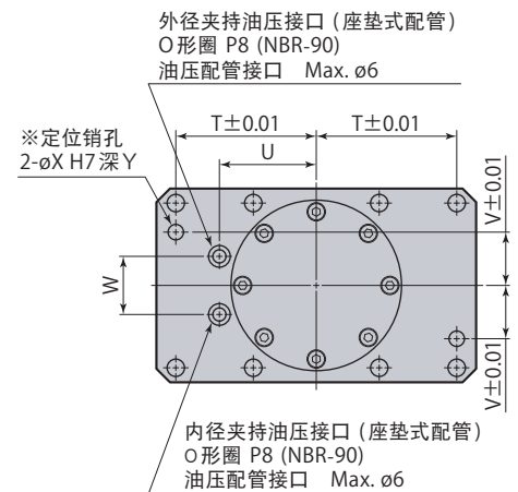
A向视图
