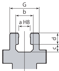
T型槽部详图
