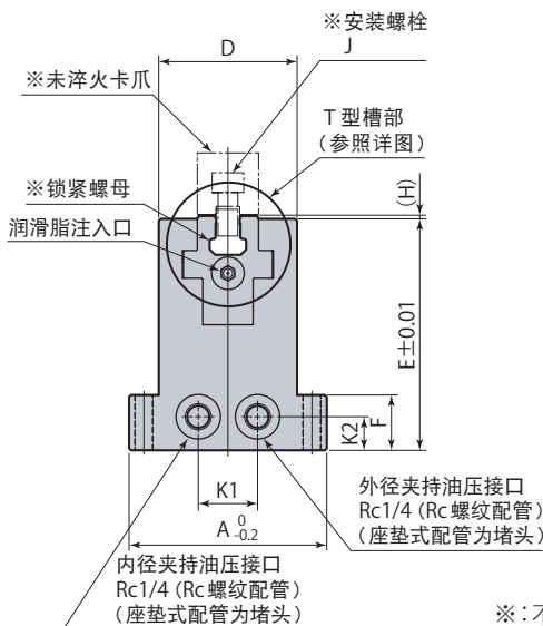
卡爪座 (锯齿节距1.5mm)
