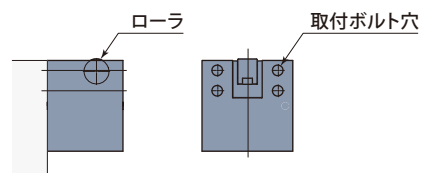
スプリングピン穴なし
