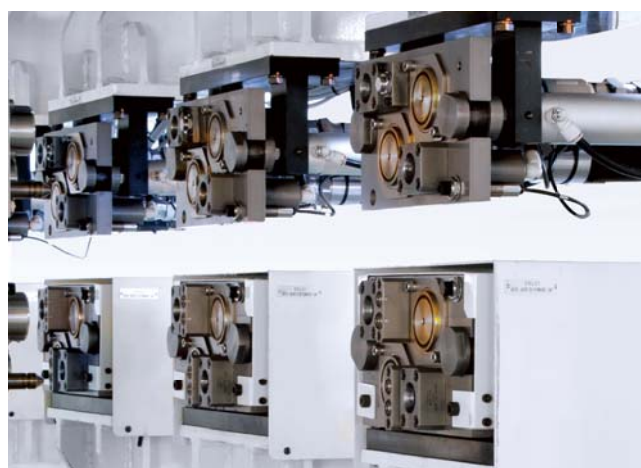
1200ton ホットプレス
