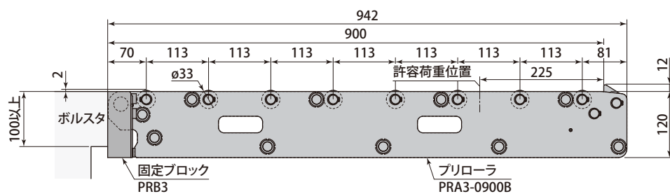
PRA3-0900B-S
