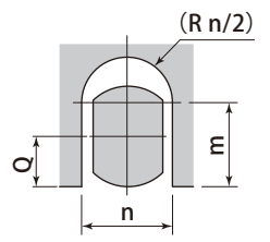
金型Uカット寸法
