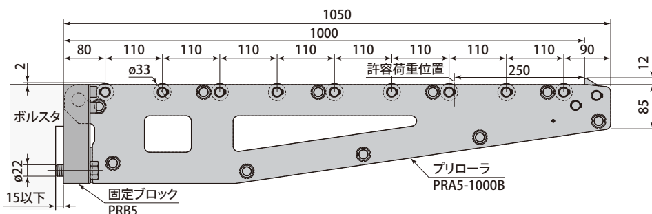
PRA5-1000B-S
