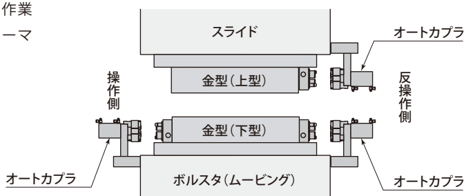
1200ton ホットプレス
