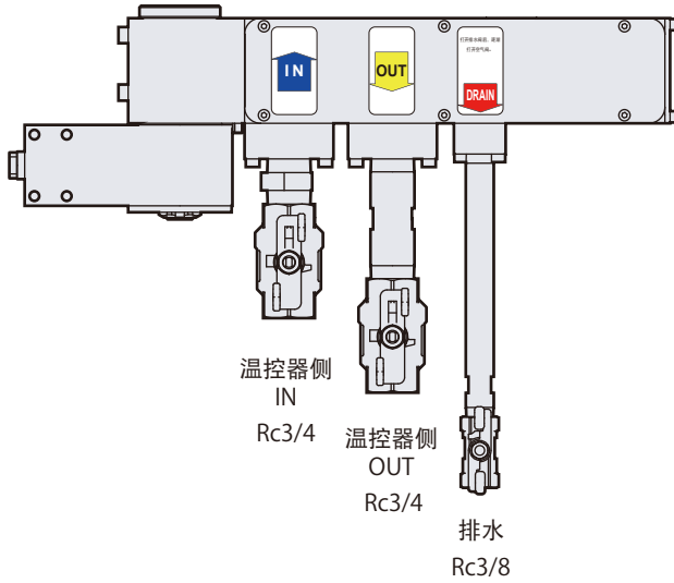
后视图
