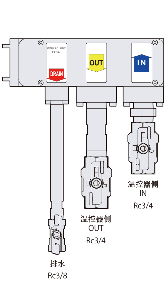
后视图
