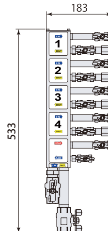
4回路(8接口) model MBA-08RHS
