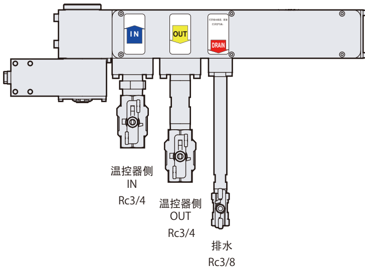
后视图
