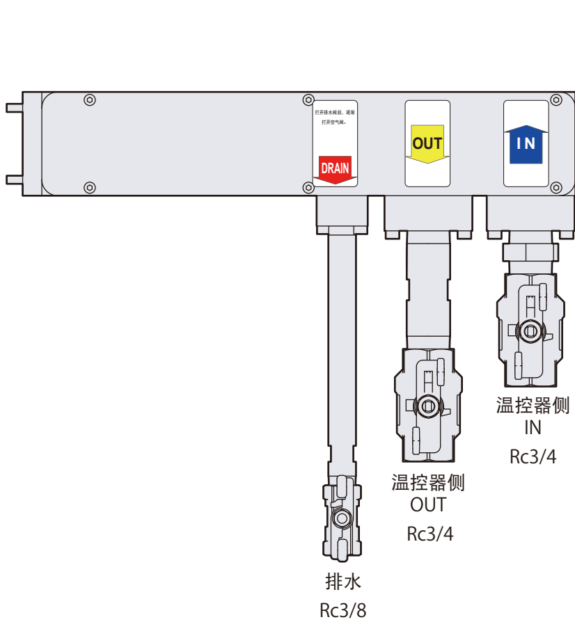
后视图
