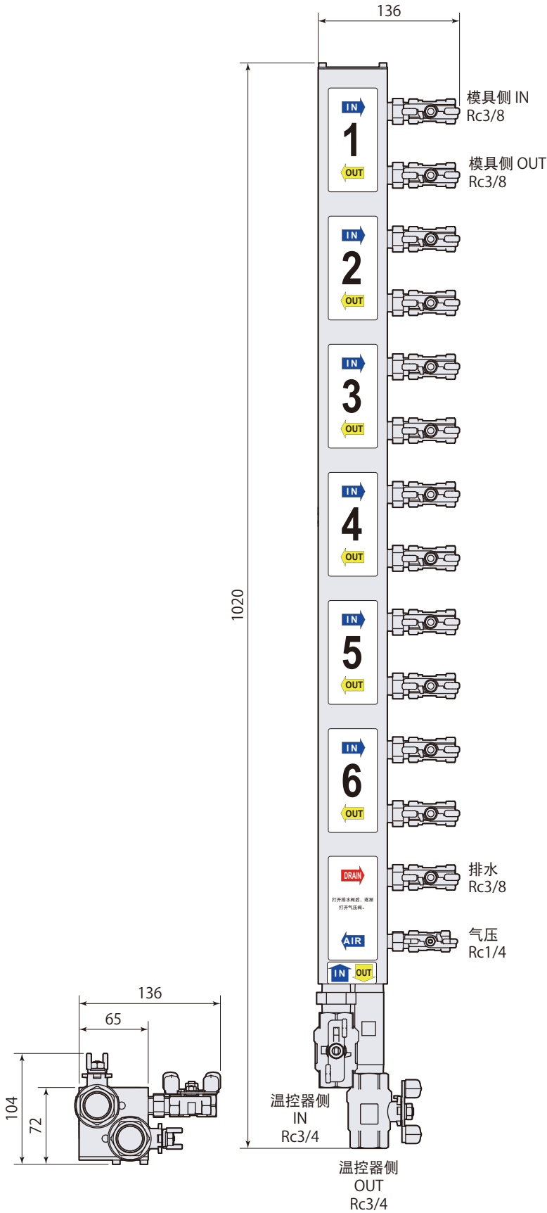
箭头视图A
