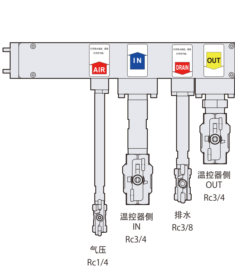
后视图
