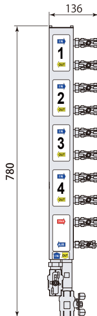
4回路(8接口) model MBA-08RH
