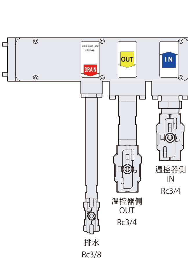
后视图
