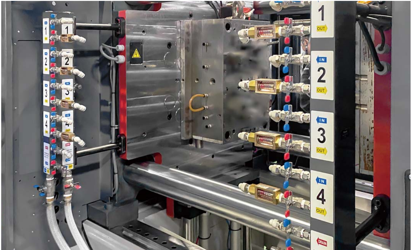
3,500 kN 注塑机 实施例 New阀座 水平型 4回路 8接口 MBA-08RH/MBA-08LH
