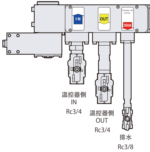
后视图
