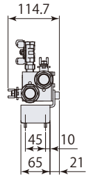
箭头视图A
