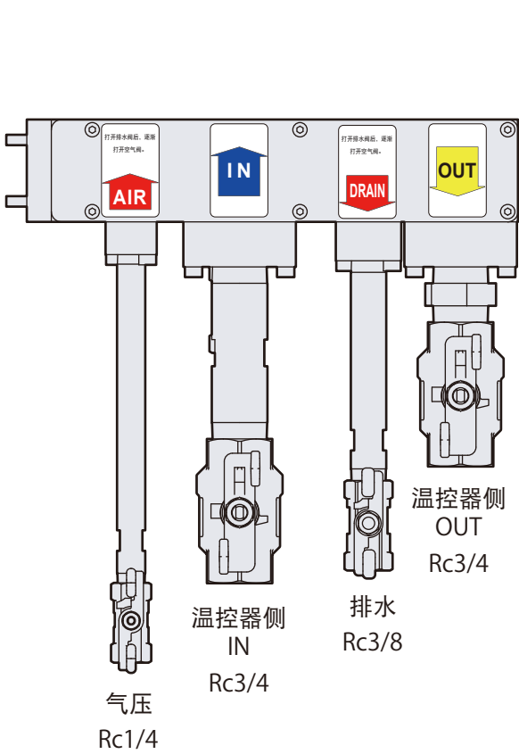
后视图
